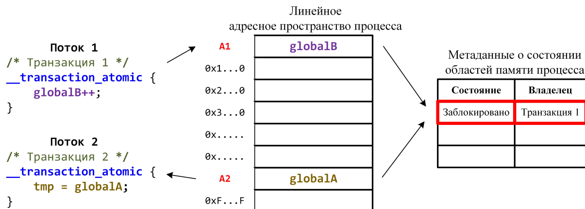
Рис. 4. Пример возникновения ложного конфликта при выполнении двух транзакций (GCC 4.8+)
