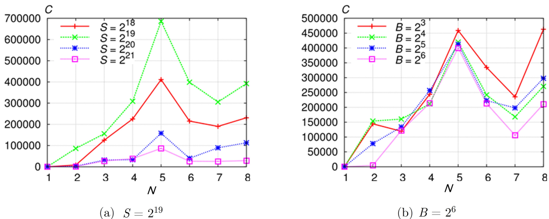
Рис. 9. Зависимость числа C ложных конфликтов от числа N потоков
