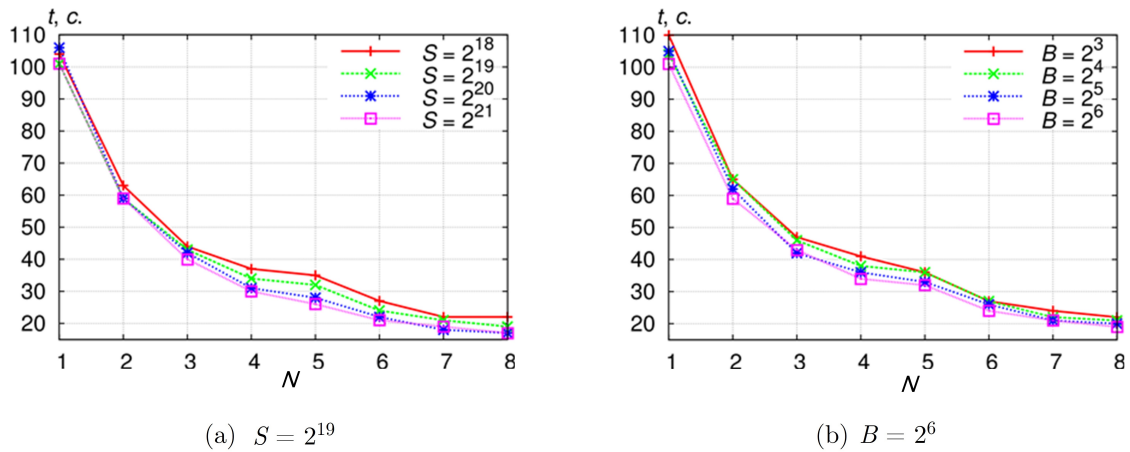
Рис. 10. Зависимость времени t выполнения теста от числа N потоков
