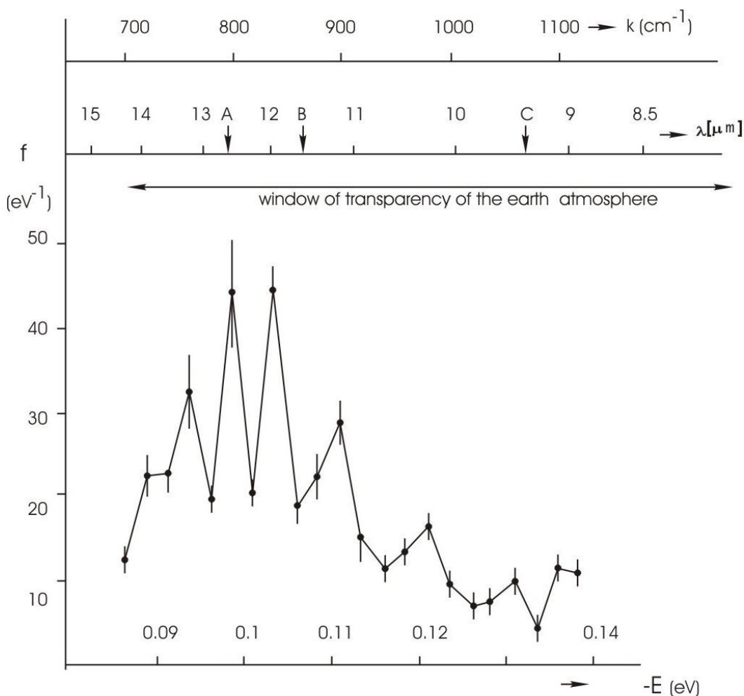
Рис. 3. Дифференциальный неравновесный энергетический спектр (ДНЭС) деионизированной воды (хим. чистота 99,99 %, pH 6,5-7,5, общая минерализация 400 мг/л, удельная электропроводность 10 мк·См/см)
