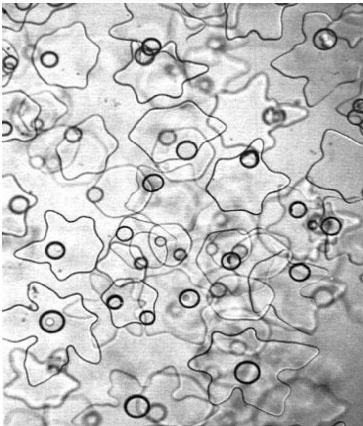
Рис. 2. Структура талой воды по данным компьютерного моделирования с «размытыми» структурами льда
