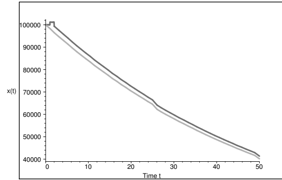
Рис. 3. Размер популяции: темная линия — кооперация, светлая — равновесие по Нэшу
