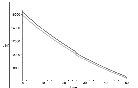
Рис. 4. Вылов первого игрока: темная линия — кооперация, светлая — равновесие по Нэшу
