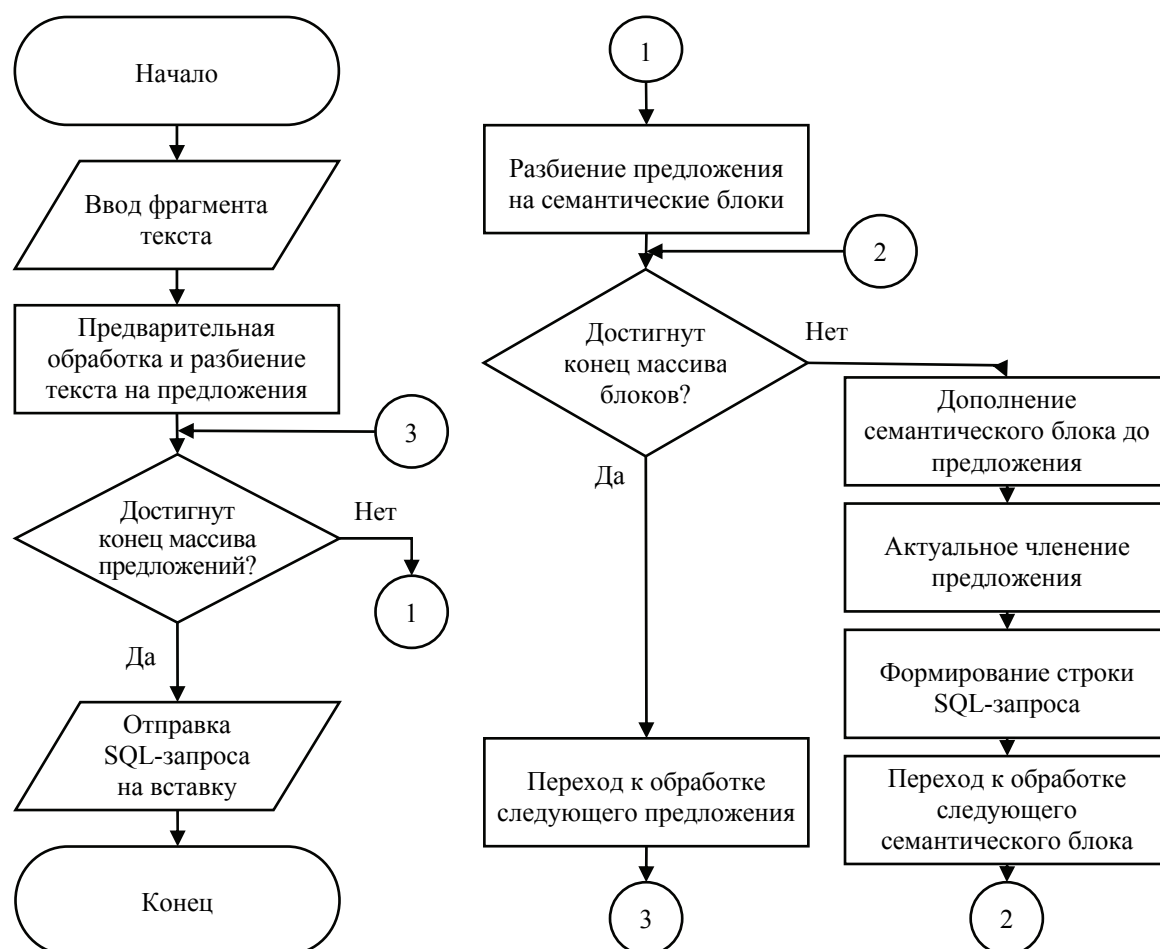
Рис. 2. Блок-схема алгоритма генерации СС
