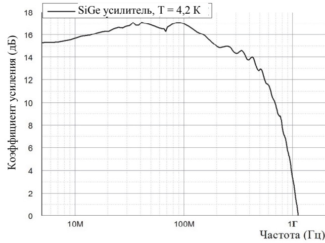
Рис. 4. Экспериментально полученный коэффициент усиления усилителя в полосе до 1,8 ГГц при температуре 4,2 К
