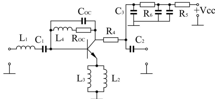
Рис. 2. Схема анализа коэффициента стабильности усилителя в СВЧ диапазоне частот
