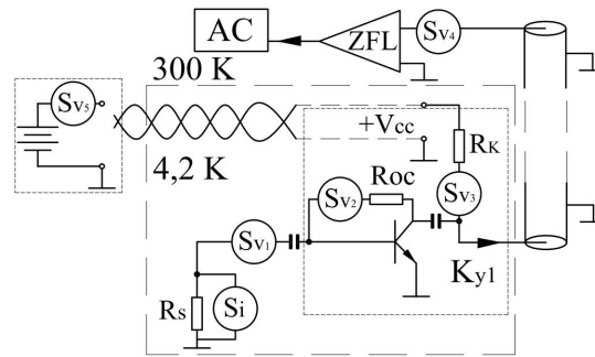
Рис. 5. Схема измерения полного шума криогенного усилителя при температуре 4,2 К
