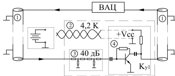
Рис. 3. Схема измерения S -параметров криогенного усилителя при температуре 4,2 К:
