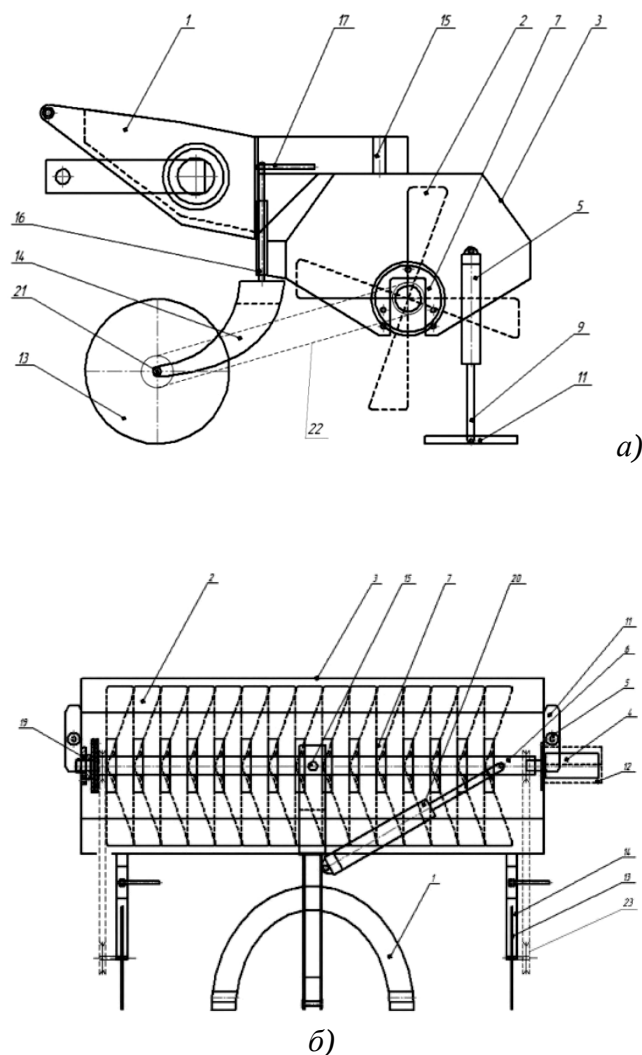
Рисунок 2 – Схема ротационного плуга а) вид сбоку; б) вид сверху
