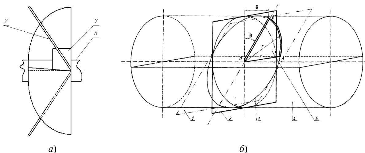
Рисунок 3 – Конструктивные параметры эллиптических лопастей
