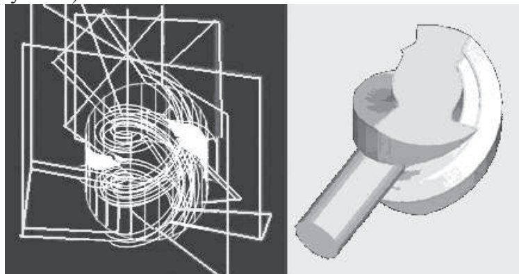
Рисунок 1. Траектория движения режущего инструмента в системе ADEM
