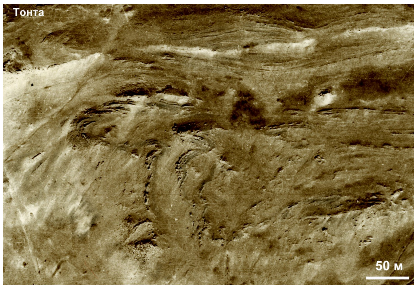
Рис. 31. а – фрагмент аэрокосмической геологической карты юго-западной части зоны Черноруд [Fedorovsky et al., 2012] – поля развития ранних складок покровного и сдвигового типов; б – аэрофотоснимок части этой территории. Хорошо видны замки крупных складок с пологими шарнирами. Интервал Тонта – Улан-Харгана.
