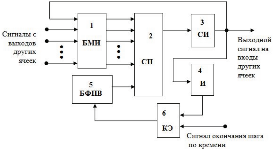
Рис. 1. Функциональная схема ячейки однородной структуры для решения дифференциальных уравнений в частных производных: 1) блок масштабных интеграторов (БМИ); 2) сумматор приращений (СП); 3) следящий интегратор (СИ); 4) интегратор (И); 5) блок формирования приращений с предыдущих шагов по времени (БФПВ); 6) ключевой элемент (КЭ)
