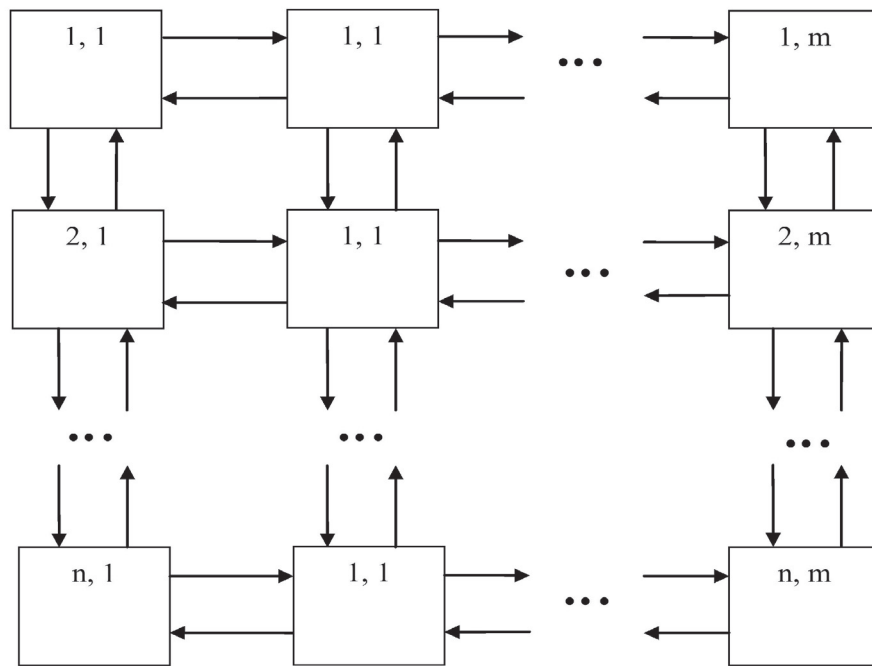
Рис. 2. Фрагмент однородной вычислительной структуры для решения дифференциальных уравнений в частных производных на разностных сетках
