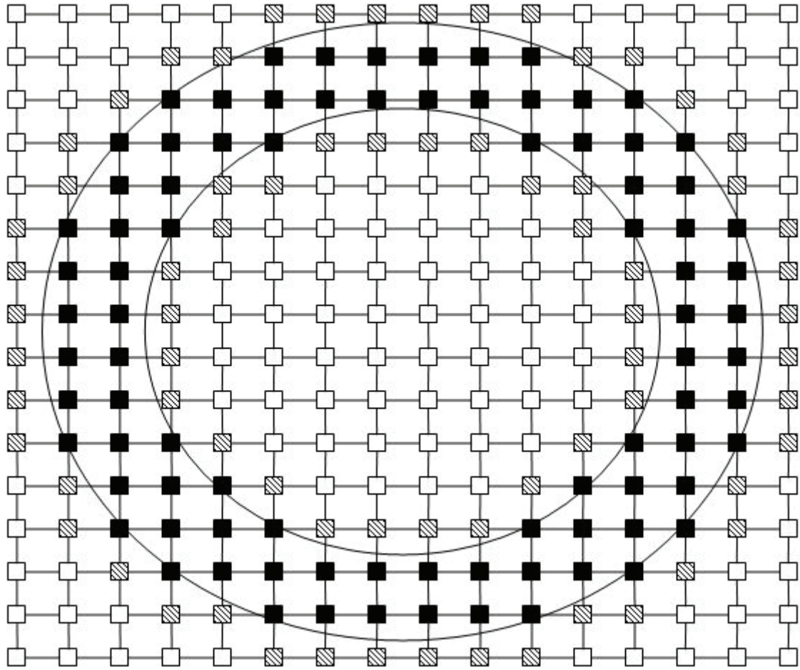
Рис. 3. Конфигурирование ячеек однородной вычислительной структуры для заданной области (показана контуром) решения дифференциальных уравнений в частных производных
