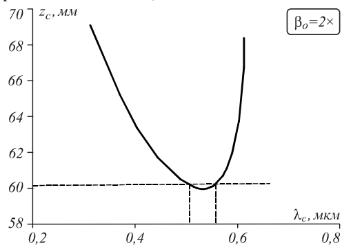
Рис. 5. Зависимость расстояния z_c от изменения рабочей длины волны \lambda_c
