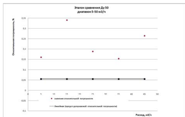
Рис. 2 - Результаты аттестации в диапазоне 5-50 м³/ч
