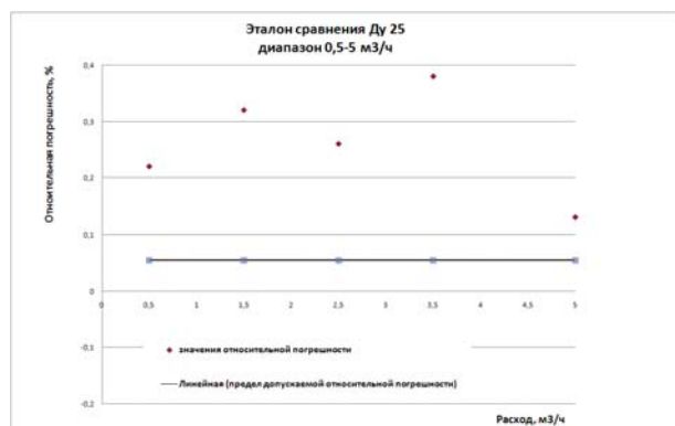
Рис. 1 - Результаты аттестации в диапазоне 0,5-5 м³/ч
