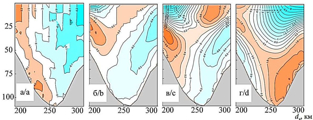
Рис. 6. Распределение меридиональной составляющей скорости течения (см/с) в северной части Татарского пролива по сезонам: а) зимой; б) весной; в) летом; г) осенью Fig. 6. Distribution of meridional component of flow velocity (cm/s) in northern part of the Tatar Strait seasonable: a) winter; b) spring; c) summer; d) autumn
