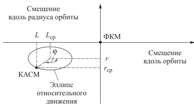
Рис. 1. К определению параметров относительного движения
