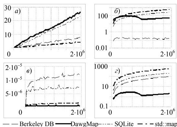
Рис. 4. Серия экспериментов для данных словарной морфологии: (а) – время построения словаря объемом n ключей ( n – абсцисса); (б) – объем памяти в Мб для формирования словаря (логарифмическая шкала); (в) – время успешного поиска в таком словаре; (г) – размер сериализованной структуры хранения в Мб (логарифмическая шкала).
