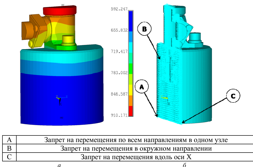
Рис. 2. Тепловое состояние в процессе огневых испытаний (а) и граничные условия в виде запрета на перемещения (б)
