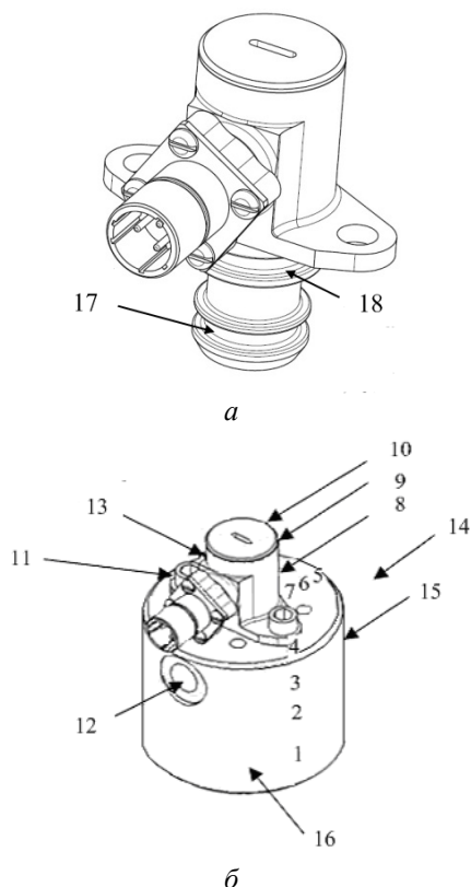
Рис. 1. Сигнализатор засорения маслофильтра (а), сборка «сигнализатор засорения – имитатор маслоагрегата» (б): 1–11 – термодатчики; 12 – подвод высокого давления; 13 – сигнализатор засорения маслофильтра; 14 – направление пламени; 15 – подвод низкого давления; 16 – имитатор маслоагрегата; 17 – канавка под нижнее уплотнительное кольцо; 18 – канавка под верхнее уплотнительное кольцо
