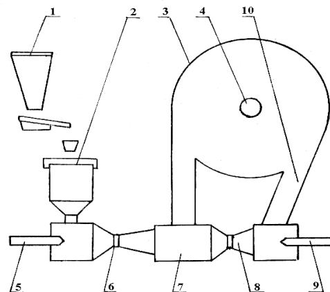
Рис. 5. Струйная мельница 1 – дозатор; 2 – бункер; 3 – сепарационная камера; 4 – выпускное отверстие; 5, 9 – сопла; 6, 8 – инжекторы; 7 – помольная камера; 10 – рукав возврата крупных частиц материала
