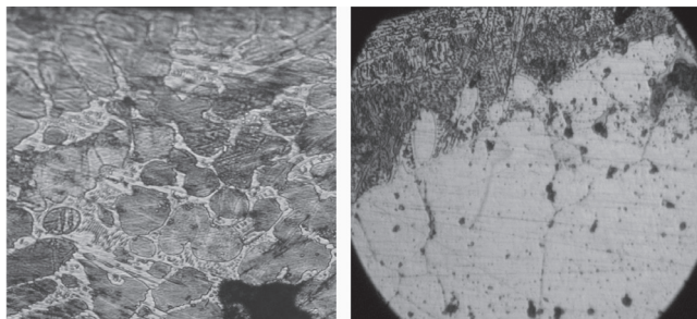
Рис. 4. Структура диффузионного слоя после ЭХТО в режиме оплавления поверхности: а – сталь 40Х; б – сталь 20. \times 500
