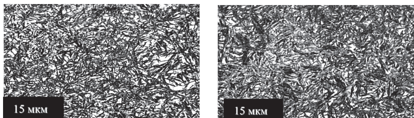
Рис. 7. Микроструктура диффузионного слоя образцов стали 65Г после термической обработки: а – закалка после нормализации; б – закалка после двух циклов. \times 1000
