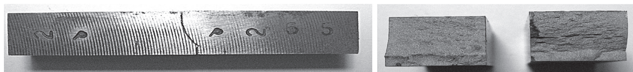
Рис. 9. Разрушение образца стали 65Г с микроструктурой мартенсита отпуса после испытания на ударную вязкость
