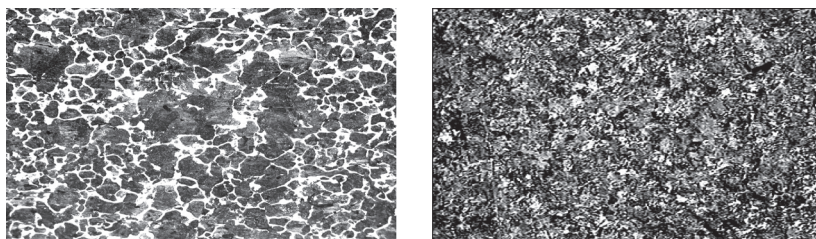
Рис. 6. Микроструктура сердцевины образца стали 65Г: а – после ХТО; б – после нормализации. \times 100
