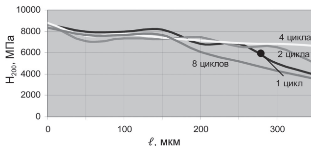
Рис. 5. Распределение микротвердости образцов стали 20 после ЭХТО с циклическим нагревом и закалкой с последующим нагревом
