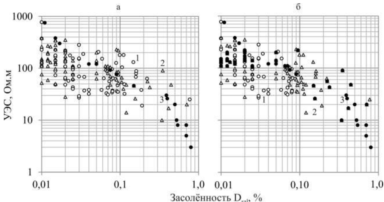
Рис. 1. Эмпирические зависимости удельного электрического сопротивления (УЭС) от показателя засоленности D_{sal} почвогрунтов СТС в полосе трасс газопроводов (а) и по литотипам почвогрунтов СТС Центрально-Якутской низменности (б). Трассы газопроводов: 1 – Таас-Тумус-Якутск; 2 – Якутск-Покровск; 3 – Якутск-Табага. Литотипы грунтов: 1 – песок; 2 – суглинок; 3 – супесь.
