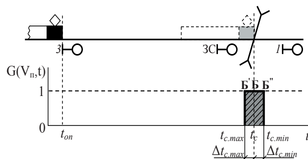
Рис. 1. Изображение функции времени возможного столкновения в зоне переезда G(V_n, t) при наличии отклонений в скорости движения поезда от графической скорости
