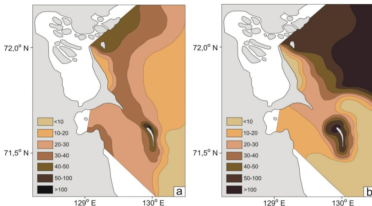
Рис. 4. Структура пространственного распределения взвешенного материала (мг/л) в водах поверхностного (а) и придонного (б) горизонтов. Сентябрь 2006 г. Безледный период
