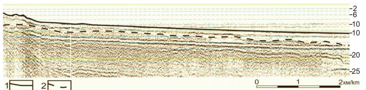
Рис. 3. Сейсмоакустический разрез через подводный береговой склон на участке от подножья окаймляющих вдольбереговых валов (неопубликованные данные В.П. Прокудина, 2007 г.)
