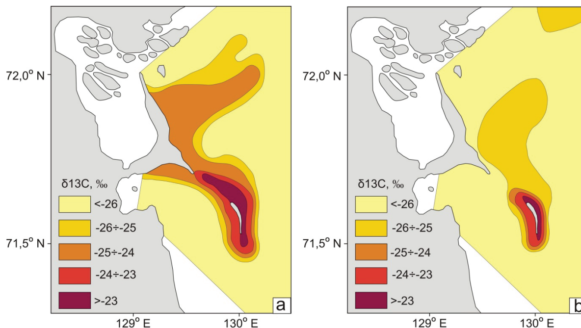
Рис. 8. Структура пространственной изменчивости изотопного состава C_{org} донных осадков в сентябре 2006 г. (a) и апреле 2007 г. (b)
