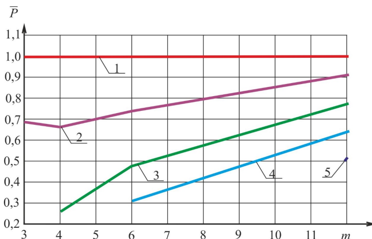
Рис. 4. Зависимость полезной мощности P многофазных машин в относительных единицах от количества работающих фаз m ; 1 – m работающих фаз; 2 – m-1 работающих фаз; 3 – m-2 работающих фаз; 4 – m-3 работающих фаз; 5 – m-4 работающих фаз
