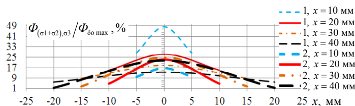
Рис. 10. Зависимости соотношения \Phi_{\sigma 3}/\Phi_{\delta 0 \max} (1) и \Phi_{(\sigma 1 + \sigma 2)}/\Phi_{\delta 0 \max} (2) в магнитной системе разнополярного генератора от x_{ВПЭГ}^{**} при x = \text{var} , Q = 40 \text{ мм} и S_{МПр} = 200 \text{ мм}^2
