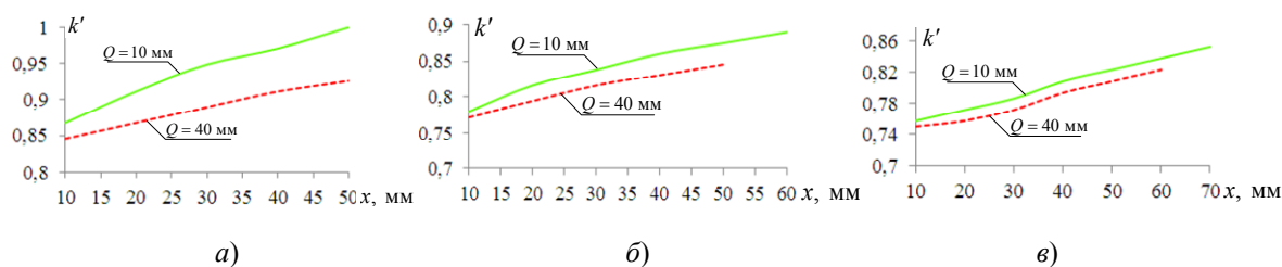
Рис. 7. Зависимости коэффициента выпучивания магнитного потока в магнитных системах однополярного 2- и 4-полюсного генераторов от величины хода подвижной части при Q = \text{var} : a - S_{\text{МПр}} = 200 \text{ мм}^2 ; б - S_{\text{МПр}} = 784 \text{ мм}^2 ; в - S_{\text{МПр}} = 1764 \text{ мм}^2
