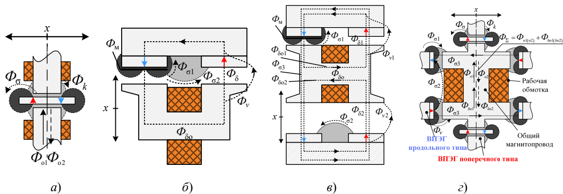
Рис. 2. Структуры магнитных систем базовых модулей ВПЭГ: а – поперечного типа; б – однополярного продольного типа; в – разнополярного продольного типа; г – комбинированного типа с общим МП
