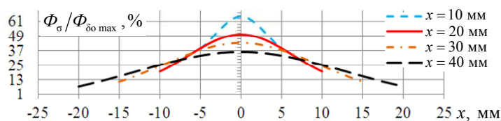
Рис. 11. Зависимости соотношений \Phi_{\sigma}/\Phi_{\delta 0 \max} в магнитной системе разнополярного генератора от x_{ВПЭГ}^{**} при x = \text{var} , Q = 40 \text{ мм} и S_{МПр} = 200 \text{ мм}^2
