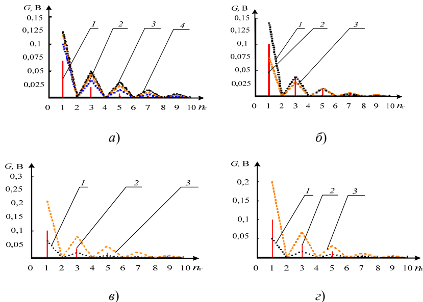
Рис. 19. Спектр ЭДС движения КГ с Ж-образным МПР: а – 1 – при x = 30 мм, S_{\text{МПР ВПЭГ попер.типа}} / S_{\text{МПР ВПЭГ прод.типа}} = 100/200 \text{ мм}^2 , f = 66,6 Гц; 2 – при x = 42 мм, S_{\text{МПР ВПЭГ попер.типа}} / S_{\text{МПР ВПЭГ прод.типа}} = 200/400 \text{ мм}^2 , f = 47,6 Гц; 3 – при x = 53 мм, S_{\text{МПР ВПЭГ попер.типа}} / S_{\text{МПР ВПЭГ прод.типа}} = 300/600 \text{ мм}^2 , f = 37,7 Гц; 4 – при x = 68 мм, S_{\text{МПР ВПЭГ попер.типа}} / S_{\text{МПР ВПЭГ прод.типа}} = 400/800 \text{ мм}^2 , f = 29,4 Гц ( v_r = 4 \text{ м/с} - \text{const} ); б – 1 – при x = 30 мм, f = 66,6 Гц; 2 – при x = 42 мм, f = 47,6 Гц; 3 – при x = 60 мм, f = 33,3 Гц ( S_{\text{МПР ВПЭГ попер.типа}} / S_{\text{МПР ВПЭГ прод.типа}} = 200 / 400 \text{ мм}^2 - \text{const} ; v_r = 4 \text{ м/с} - \text{const} ); в – 1 – при S_{\text{МПР ВПЭГ попер.типа}} / S_{\text{МПР ВПЭГ прод.типа}} = 100/200 \text{ мм}^2 ; 2 – при S_{\text{МПР ВПЭГ попер.типа}} / S_{\text{МПР ВПЭГ прод.типа}} = 200/400 \text{ мм}^2 ; 3 – при S_{\text{МПР ВПЭГ попер.типа}} / S_{\text{МПР ВПЭГ прод.типа}} = 400/800 \text{ мм}^2 ( x = 42 \text{ мм} - \text{const} ; f = 47,6 \text{ Гц} - \text{const} ; v_r = 4 \text{ м/с} - \text{const} ); г – 1 – при f = 23,8 Гц, v_r = 2 \text{ м/с} ; 2 – при f = 47,6 Гц, v_r = 4 \text{ м/с} ; 3 – при f = 95,4 Гц, v_r = 8 \text{ м/с} ( x = 42 \text{ мм} - \text{const} ; S_{\text{МПР ВПЭГ попер.типа}} / S_{\text{МПР ВПЭГ прод.типа}} = 200/400 \text{ мм}^2 - \text{const} )
