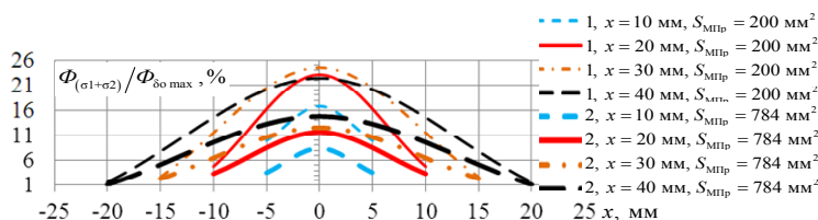
Рис. 16. Зависимости соотношений \Phi_{(\sigma 1+\sigma 2)}/\Phi_{\delta o \max} в магнитной системе разнополярного генератора от x_{\text{ВПЭГ}}^{**} при x = \text{var} , Q = 40 мм, S_{\text{МПр}} = 200 мм 2 и S_{\text{МПр}} = 784 мм 2
