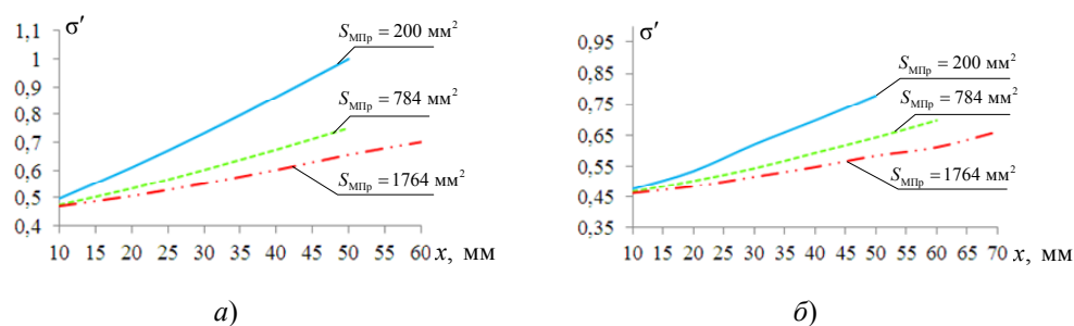
Рис. 6. Зависимости коэффициента рассеяния магнитного потока в магнитных системах однополярного 2- и 4-полюсного генераторов от величины хода подвижной части при S_{\text{МПр}} = \text{var} : a - Q = 10 \text{ мм} ; б - Q = 40 \text{ мм}
