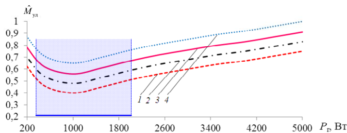
Рис. 23. Зависимости удельной массы ВПЭГ продольного типа от P_r : 1 – 10 мм; 2 – 20 мм; 3 – 30 мм; 4 – 40 мм
