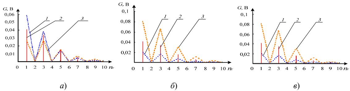
Рис. 18. Спектр ЭДС движения разнополярного генератора продольного типа: а – 1 – при x = 30 мм, f = 66,6 Гц; 2 – при x = 42 мм, f = 47,7 Гц; 3 – при x = 60 мм, f = 33,3 Гц ( S_{\text{МПР}} = 200 \text{ мм}^2 - \text{const} ; v_r = 4 \text{ м/с} - \text{const} ); б – 1 – при S_{\text{МПР}} = 100 \text{ мм}^2 ; 2 – при S_{\text{МПР}} = 200 \text{ мм}^2 ; 3 – при S_{\text{МПР}} = 400 \text{ мм}^2 ( x = 42 \text{ мм} - \text{const} ; f = 47,6 \text{ Гц} - \text{const} ; v_r = 4 \text{ м/с} - \text{const} ); в – 1 – при f = 23,8 Гц, v_r = 2 \text{ м/с} ; 2 – при f = 47,7 Гц, v_r = 4 \text{ м/с} ; 3 – при f = 95,4 Гц, v_r = 8 \text{ м/с} ( x = 42 \text{ мм} - \text{const} ; S_{\text{МПР}} = 200 \text{ мм}^2 - \text{const} )
