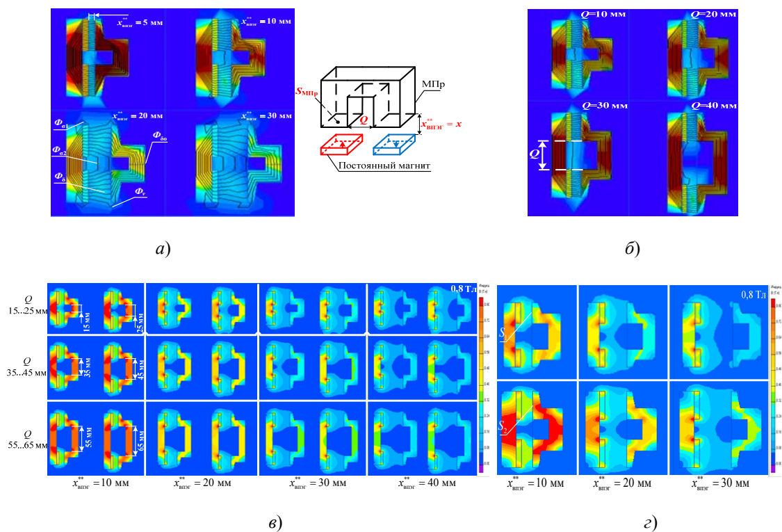
Рис. 3. Двухмерные КЭ модели МП
