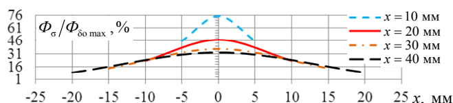
Рис. 14. Зависимости соотношений \Phi_{\sigma}/\Phi_{\delta 0 \text{ max}} в магнитной системе разнополярного генератора от x_{\text{ВПЭГ}}^{**} при x = \text{var} , Q = 40 \text{ мм} и S_{\text{МПр}} = 784 \text{ мм}^2
