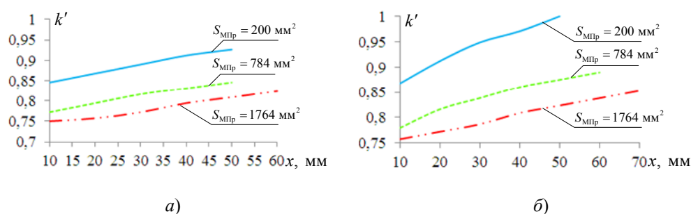
Рис. 8. Зависимости коэффициента выпучивания магнитного потока в магнитных системах однополярного 2- и 4-полюсного ВПЭГ от величины хода подвижной части при S_{\text{МПр}} = \text{var} : a - Q = 10 \text{ мм} ; б - Q = 40 \text{ мм}
