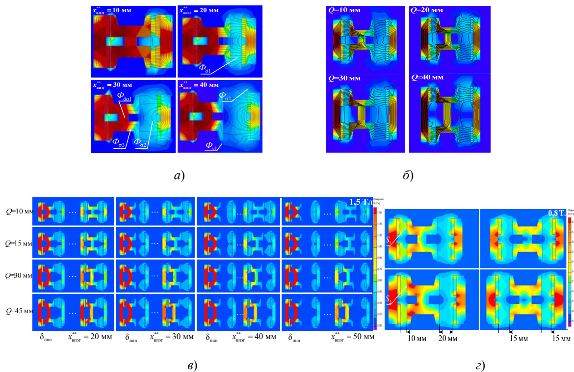
Рис. 4. Двухмерные КЭ модели МП в разнополярном ВПЭГ продольного типа:
