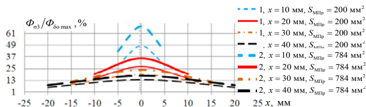
Рис. 15. Зависимости соотношений \Phi_{\sigma 3}/\Phi_{\delta o \max} в магнитной системе разнополярного генератора от x_{\text{ВПЭГ}}^{**} при x = \text{var} , Q = 40 мм, S_{\text{МПр}} = 200 мм 2 и S_{\text{МПр}} = 784 мм 2
