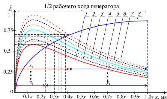
Рис. 20. Зависимости ЭДС движения ВПЭГ продольного и поперечного типов от x_{\text{ВПЭГ}}^{**} :
