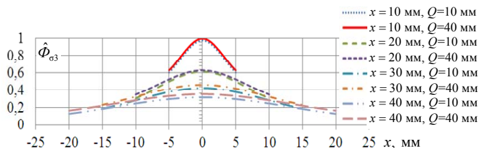
Рис. 12. Зависимости сквозного потока рассеяния магнитной системы разнополярного генератора от x_{\text{ВПЭГ}}^{**} при x = \text{var} , Q = \text{var} и S_{\text{МПр}} = 784 \text{ мм}^2
