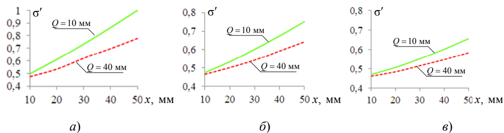
Рис. 5. Зависимости коэффициента рассеяния магнитного потока в магнитных системах однополярного 2- и 4-полюсного генераторов от величины хода подвижной части при Q = \text{var} : a - S_{\text{МПр}} = 200 \text{ мм}^2 ; б - S_{\text{МПр}} = 784 \text{ мм}^2 ; в - S_{\text{МПр}} = 1764 \text{ мм}^2
