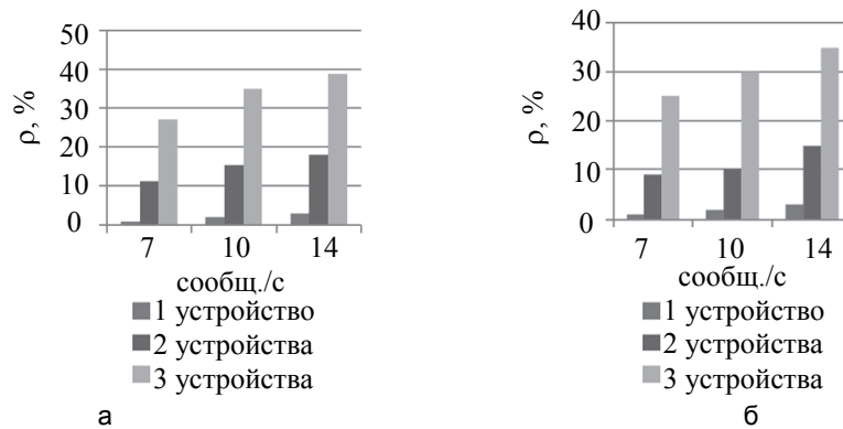
Рис. 4. Потери сообщений p (%) в зависимости от количества устройств, частоты передачи (7, 10, 14 сообщений в секунду) широковещательных команд типа: запрос информации о параметрах устройств AT+N (а); запрос идентификаторов взаимодействующих соседей AT+SN:00 (б)
