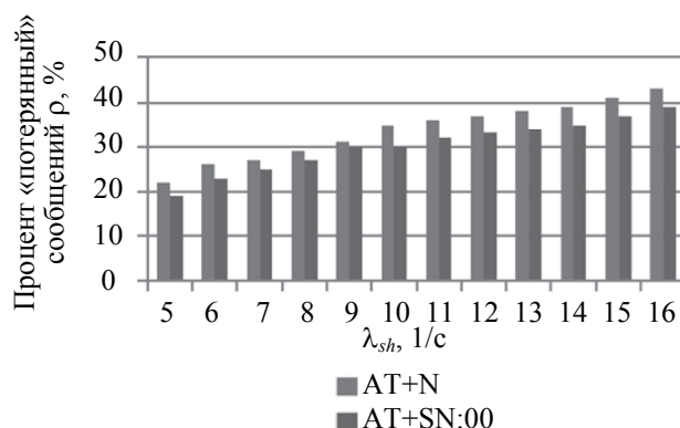
Рис. 6. Экспериментальные значения потерь сообщений p (%) для k=3
