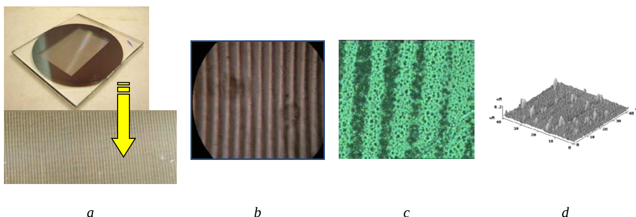
Рис. 1. Разные рельефы поверхности, получаемые методами: а – фотолитографии с шириной бороздок 10, 20 и 40 микрометра; б – методом полива и центрифугированием водного 8 %-го раствора поливинилового спирта (ПВС) с последующим натиранием хлопчатобумажной тканью; в – голографическим методом при использовании схемы четырехволнового смешения лазерных лучей на длине волны 532 нм с записью решетки на полиимидном покрытии на пространственной частоте 100 \text{ мм}^{-1} ; д – методом лазерного ориентированного осаждения УНТ на поверхность проводящего ИТО-контакта при использовании \text{CO}_2 -лазера на длине волны 10,6 микрометров с последующей обработкой поверхностной электромагнитной волной
