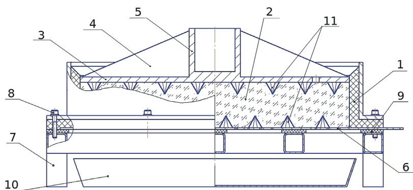
Рис. 1. Устройство дегидрататора:
