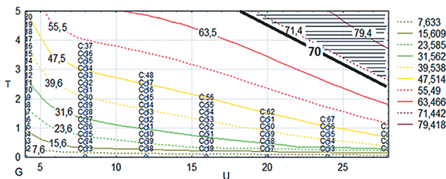
Рис. 2. Двумерное сечение модели влияния напряжения между электродами U(B) и длительности обработки T (ч) на количество отведенной влаги G (кг)
