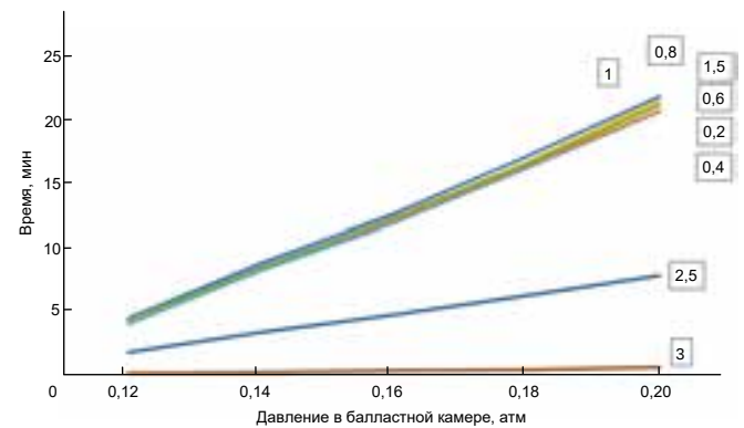
Рисунок 3. График изменения проницаемости для известняка. Цифры в квадратах обозначают давление пресса в МПа [5]. Figure 3. Permeability graph for limestone. The numbers in squares indicate the pressure of the press in MPa [5].
