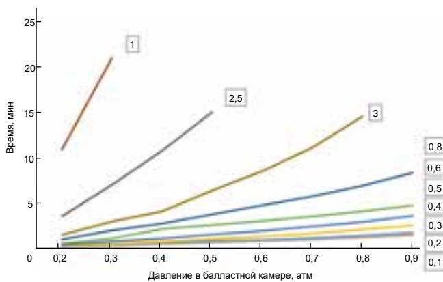
Рисунок 2. График изменения проницаемости для породы андезит-базальтового состава. Цифры в квадратах обозначают давление пресса в МПа [5]. Figure 2. Graph of change in permeability for andesite-basalt composition. The numbers in squares indicate the pressure of the press in MPa [5].
