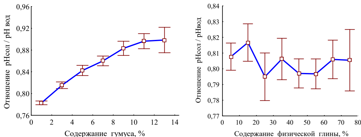
Рис. 5. Влияние содержания в почве гумуса и глины на величину отношения pH_{sol} / pH_{вод}
