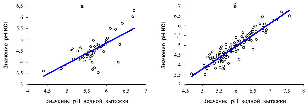
Рис. 3. Характер связи между значениями pH водной и солевой вытяжек, оцененными для гумусово-элювиального горизонта дерново-подзолистых (а) и бурых лесных (б) почв Марийского Заволжья
