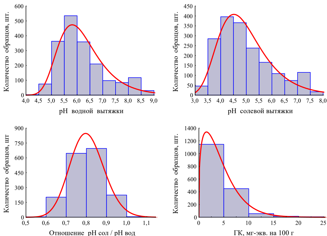
Рис. 1. Характер распределения образцов почвы в выборке по значениям показателей её кислотности
