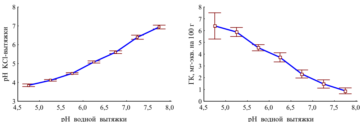
Рис. 2. Характер связи между разными показателями кислотности почвы в выборке
