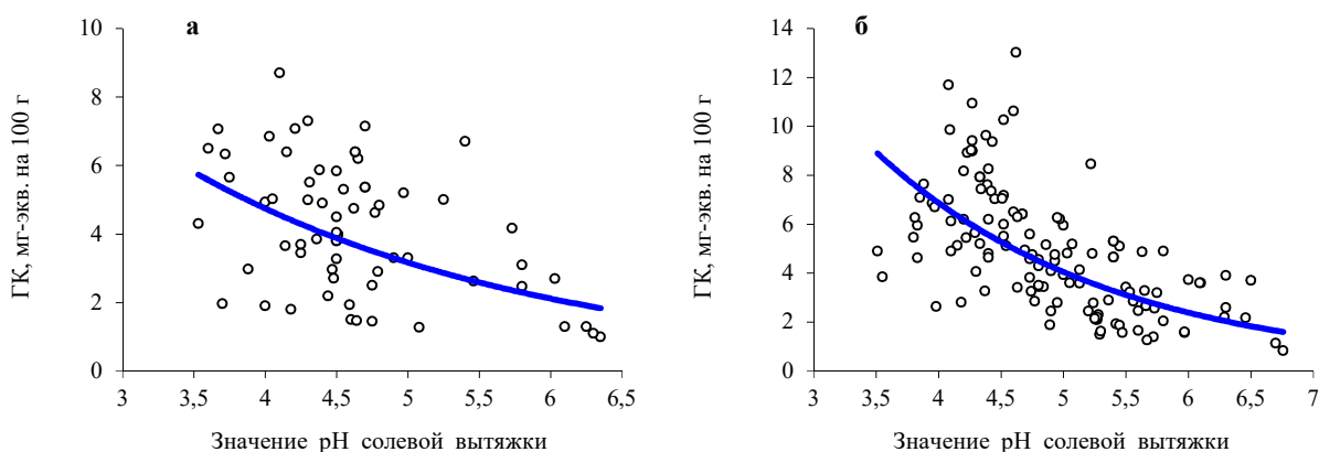
Рис. 4. Характер связи между значениями pH солевой вытяжки и гидролитической кислотности гумусово-элювиального горизонта дерново-подзолистых (а) и бурых лесных (б) почв Марийского Заволжья
