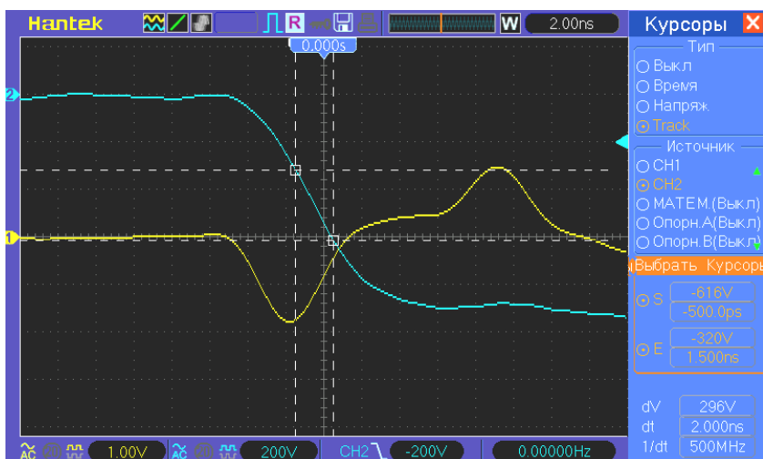
Рис. 3. Осциллограмма для диода 5ДШ402А9: форма волны напряжения – голубая (верхняя), форма тока – желтая (нижняя). Амплитуда импульса обратного напряжения, приложенного через диод V_A=900 В. dV/dt=148 В/нс
