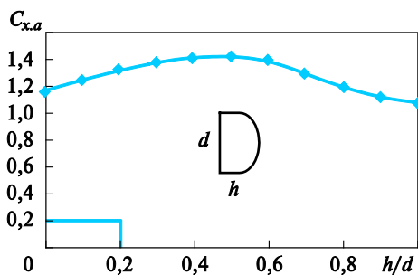
Рис. 2. Зависимость коэффициента лобового сопротивления для жестких тел от соотношения диаметра входного отверстия к высоте тела
