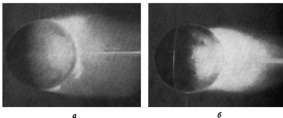
Рис. 15. Затягивание отрыва на поверхности сферы за счет применения турбулизатора: а — обычная сфера; б — сфера с проволоочным кольцом в передней части
