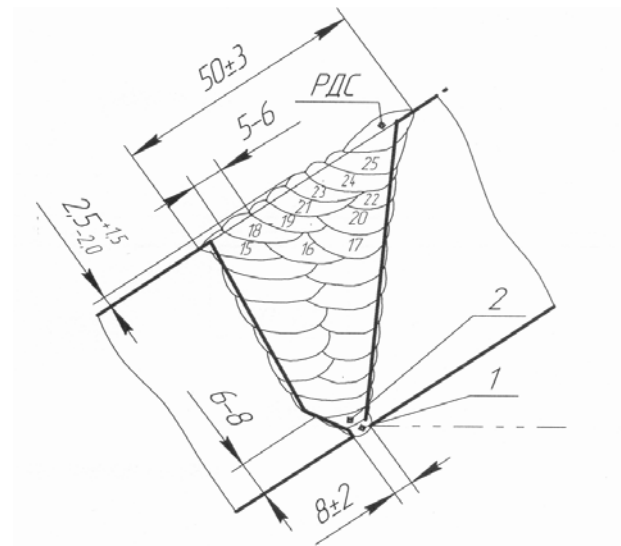
Рис. 3. Сварное соединение стали 10ХСНД толщиной 50 мм. Автоматическая сварка проволокой Св-10НМА под флюсом АН-47
