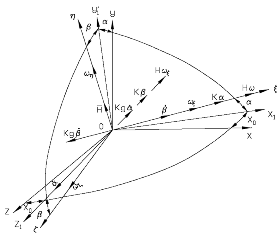
Рисунок 2 – Система координат, связанная с векторами моментов сил и кинетического момента гироскопа
