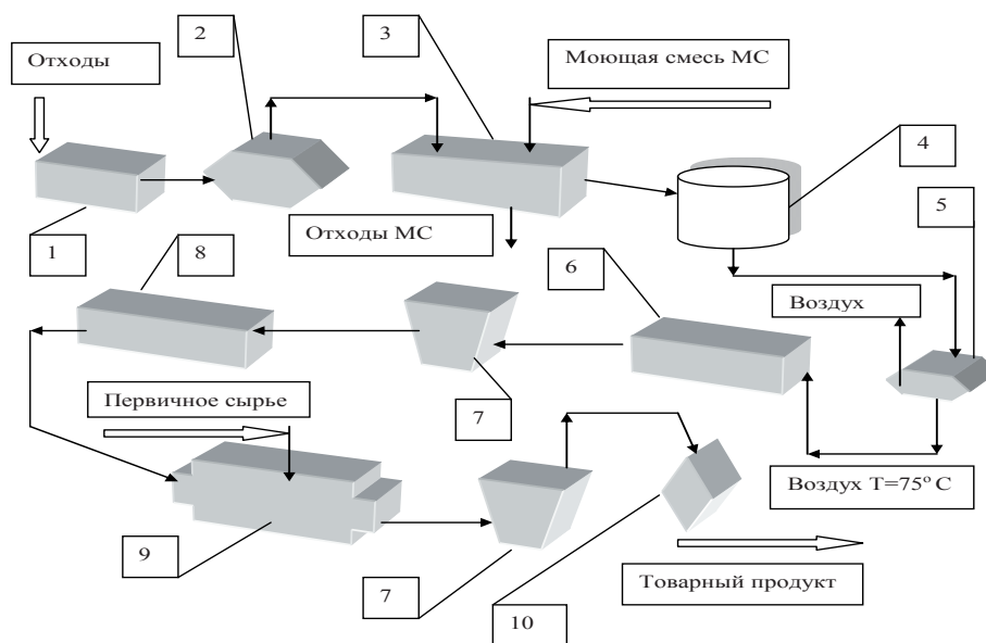
Рис. 2. Схема утилизации отходов упаковочной пленки. 1 — узел сортировки отходов; 2 — дробилка; 3 — моечная машина; 4 — центрифуга; 5 — сушилка; 6 — питатель; 7 — экструзионный пресс; 8 — гранулятор; 9 — смеситель; 10 — пленочный агрегат
