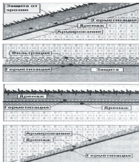
Рис. 4. Примеры применения синтетических полимерных покрытий («геосинтетики») при сооружении полигонов ТБО
