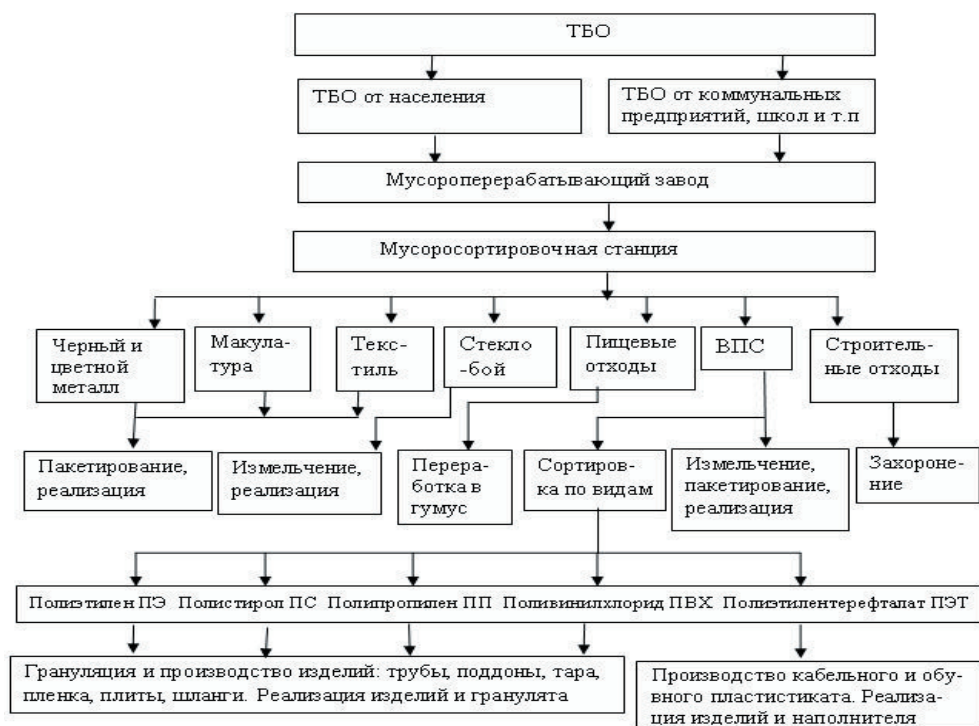
Рис. 3. Принципиальная схема переработки ТБО с утилизацией ценных компонентов и рекуперацией энергии
