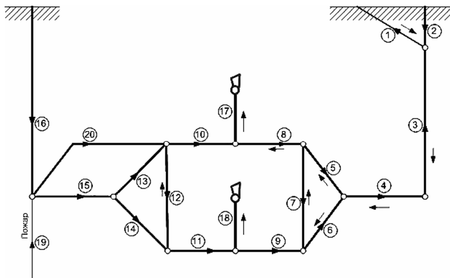
Рис. 4. Распределение газового облака в выработках (ветвях) к 17-й минуте
