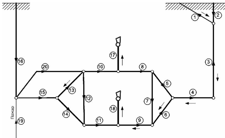
Рис. 3. Распределение газового облака в выработках (ветвях) к концу второй минуты
