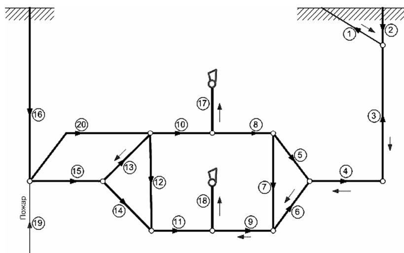
Рис. 2. Начальный момент реверсии общерудничной вентиляционной струи (ГВУ еще не запущена в реверсивный режим)
