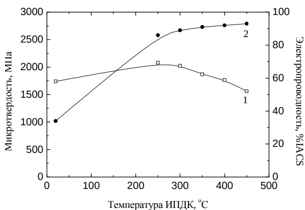
Рис. 6. Зависимость микротвердости (1) и электропроводности (2) УМЗ образцов медного сплава от температуры ИПДК
