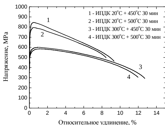
Рис. 9. Диаграммы растяжения медного сплава в УМЗ состоянии после ИПДК 20 и 300 °С с последующим старением при температурах 450 и 500 °С с выдержкой 30 минут
