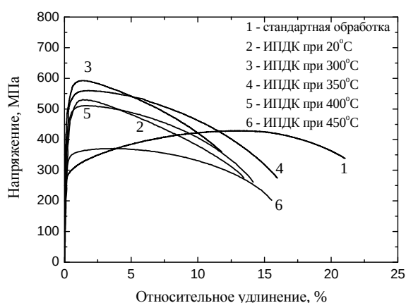
Рис. 8. Диаграммы растяжения медного сплава после ИПДК при различных температурах
