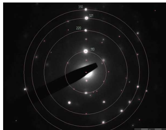
Рис. 5. Электронограмма, снятая с частиц, наблюдающихся в медном сплаве Cu-Cr, подвергнутого ИПДК при температуре 300 °С
