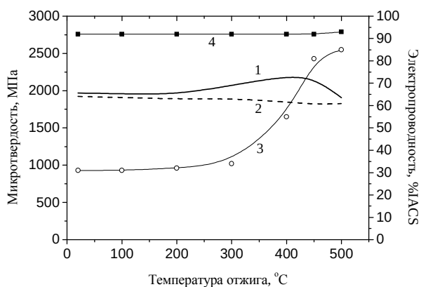
Рис. 7. Зависимость микротвердости (1, 2) и электропроводности (3, 4) УМЗ образцов медного сплава от температуры дополнительной термообработки: (1, 3) ИПДК при 20 °C; (2, 4) ИПДК при 300 °C
