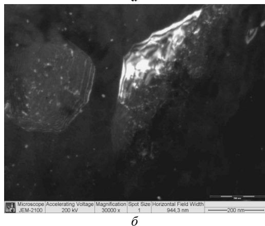
Рис. 4. Структура сплава Cu-Cr, подвергнутого ИПДК при температуре 300 °С
