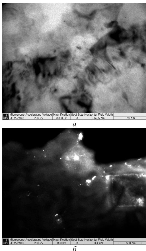
Рис. 2. Микроструктура сплава Cu-Cr, подвергнутого ИПДК при 20 °С, и дополнительному отжигу при 500 °С: а – светлопольное изображение; б – темнопольное изображение
