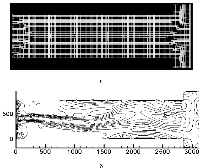
Рис. 1. Моделирование топки котла UT-L18:
