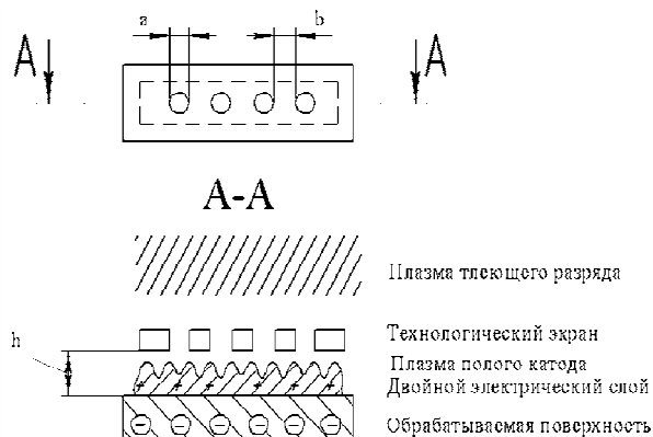
Рис. 1. Схема формирования тлеющего разряда с эффектом полого катода
