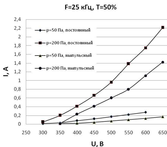
Рис. 3. Зависимость ВАХ от давления p при импульсном и постоянном режиме
