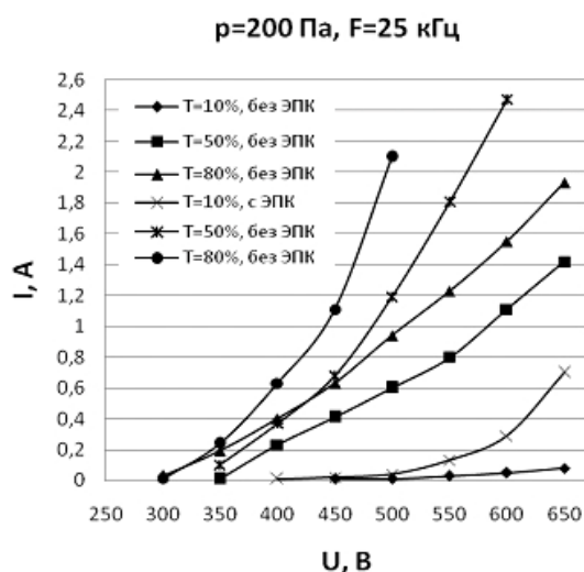
Рис. 4. Зависимость ВАХ с ЭПК и без ЭПК при импульсном режиме от скважности T
