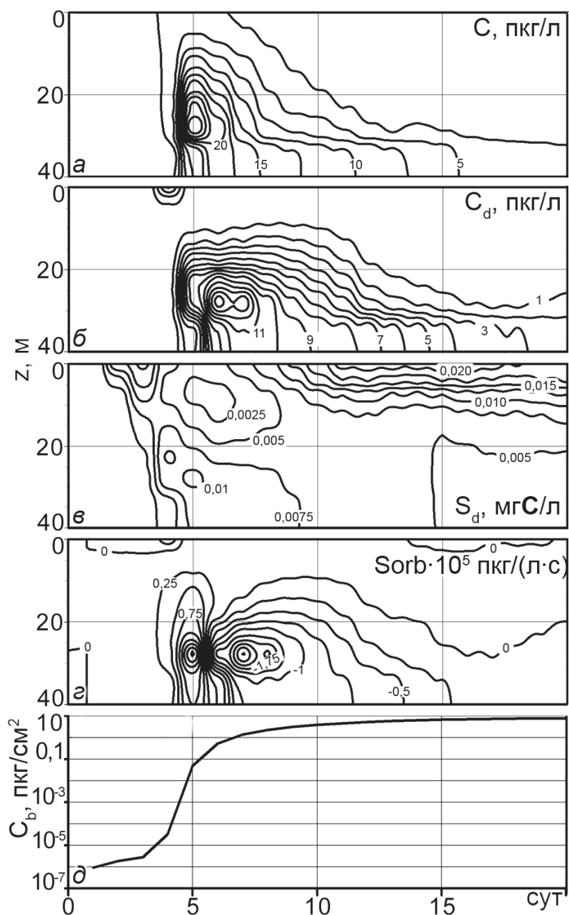
Р и с. 5. Диаграммы Хофмеллера для станции А: концентрации ПХБ в растворе (а), ПХБ на детрите (б), детрита (в); сорбционное слагаемое функции мощности источников (г); зависимость концентрации ПХБ в верхнем слое донных осадков от времени (д). Результаты численного эксперимента
