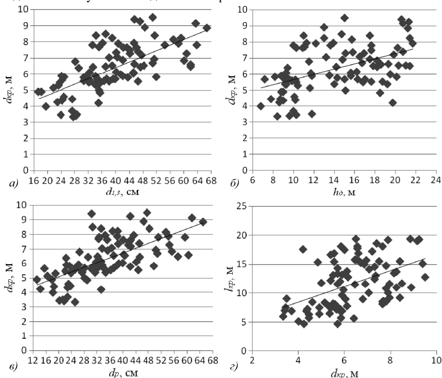
Рис. 2. Залежність діаметра крони від діаметра на висоті грудей (а), висоти дерева (б), діаметра розгалуження дерева (в) та протяжності крони (г)
