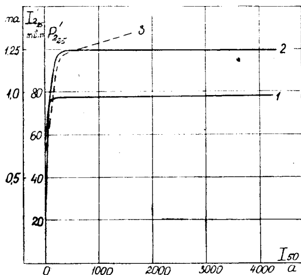
Рис. 4. Кривая 1 — зависимость вторичной мощности на частоте 25 герц фильтра нулевой последовательности от рабочего тока генератора; кривая 2 — то же для вторичного тока 25 герц; кривая 3 — расчет; кривая 4 — эксперимент
