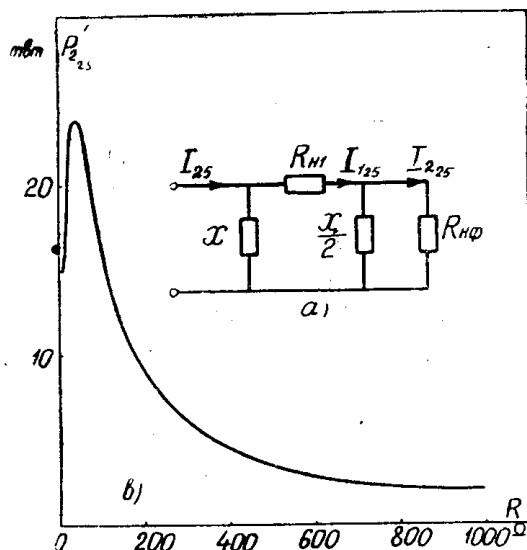
Рис. 3. а) Расчетная схема замещения 3-трансформаторного фильтра, б) зависимость вторичной мощности от сопротивления нагрузки 3-трансформаторного фильтра
