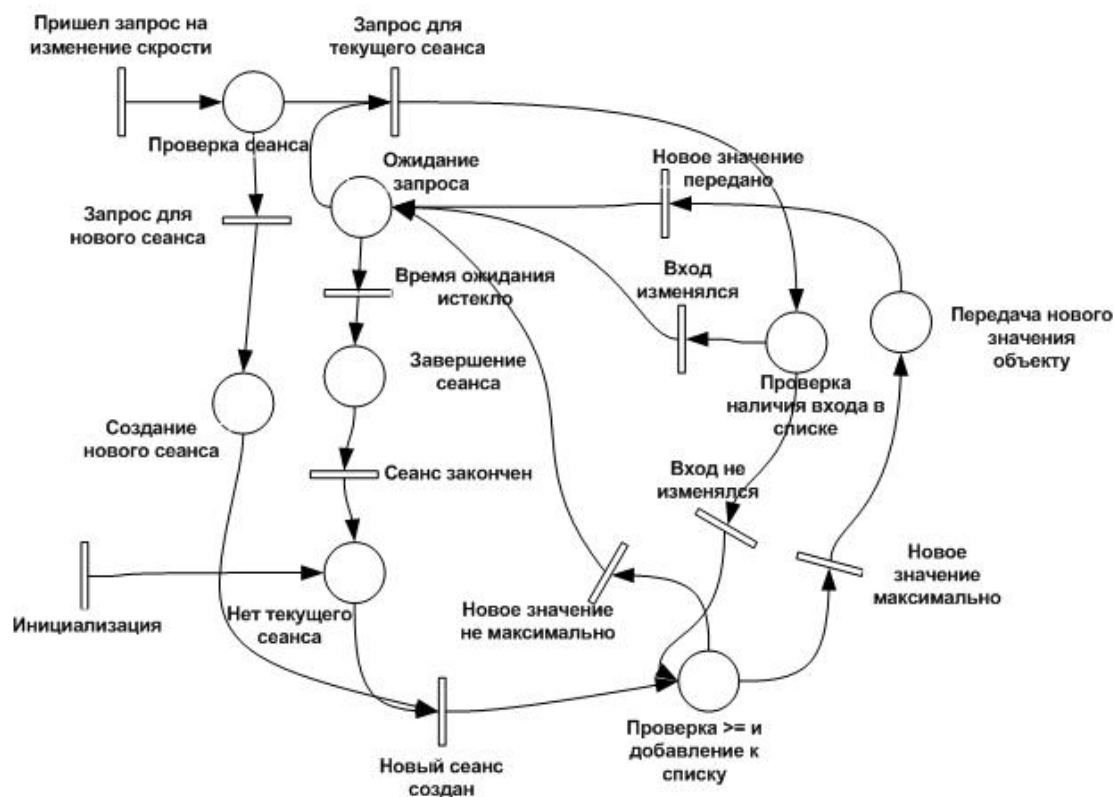
Рис. 2 — Сеть Петри, описывающая алгоритм подстройки скоростей потоков
