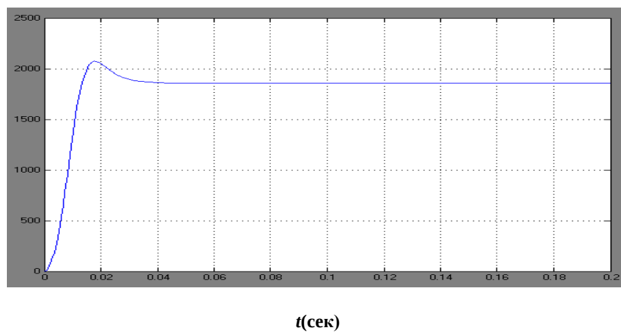
Рис. 4. Установление значений напора H(t)
