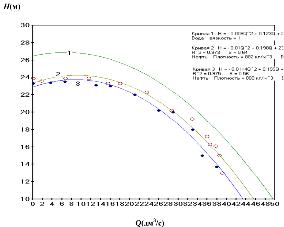
Рис. 7. Зависимость H = f(Q) для нефтей плотностью \rho = 882 \text{ кг/м}^3 (кривая 2) и \rho = 888 \text{ кг/м}^3 (кривая 3). Кривая 1 – расчетная зависимость для воды
