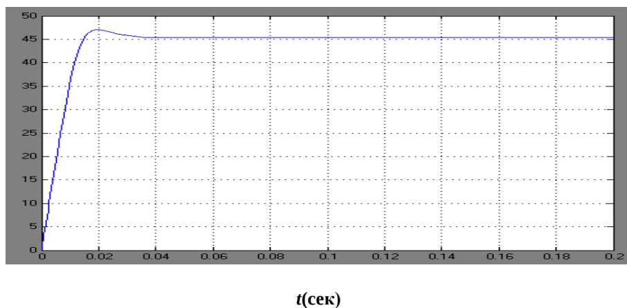
Рис. 6. Установление значений скорости ротора ПЭД \omega(t)
