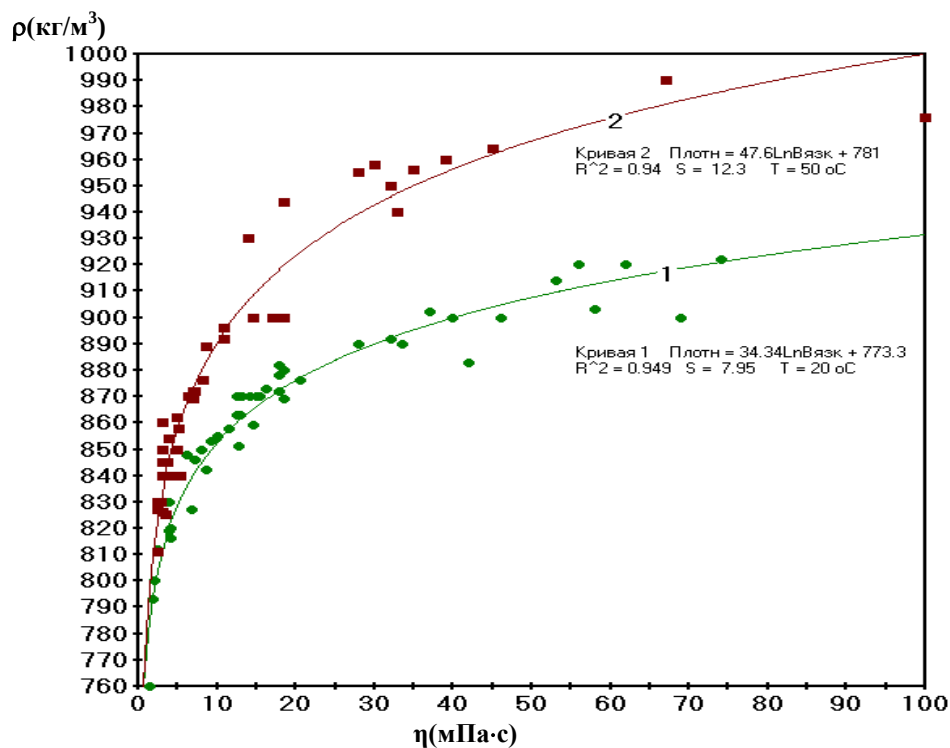
Рис.1. Зависимость между плотностью \rho и динамической вязкостью \eta для температур: 1 – (20±1)°C; 2 – (50±1)°C
