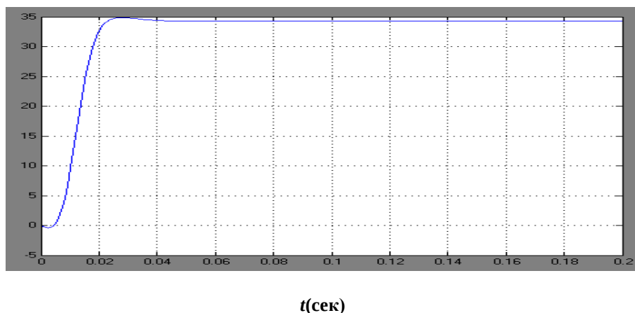
Рис. 5. Установление значений производительности Q(t)
