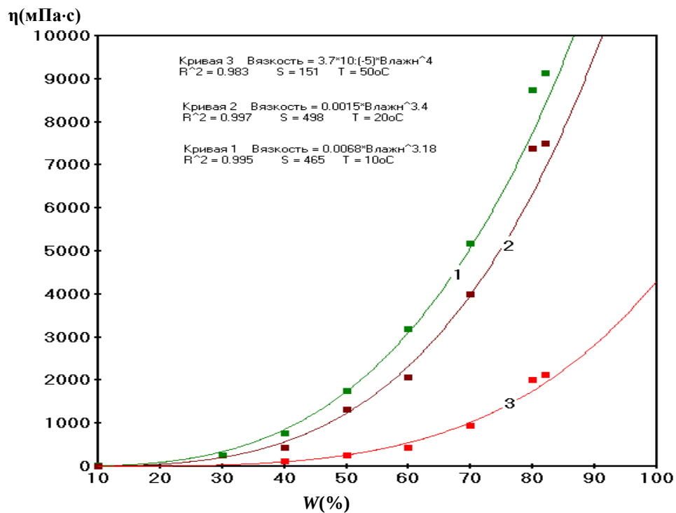
Рис.2. Зависимость вязкости \eta в водонефтяных эмульсиях от концентрации воды W для температур: 1 – 10 °C; 2 – 20 °C; 3 – 50 °C
