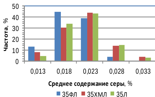
Рис. 1. Распределение плавов сталей по содержанию серы
