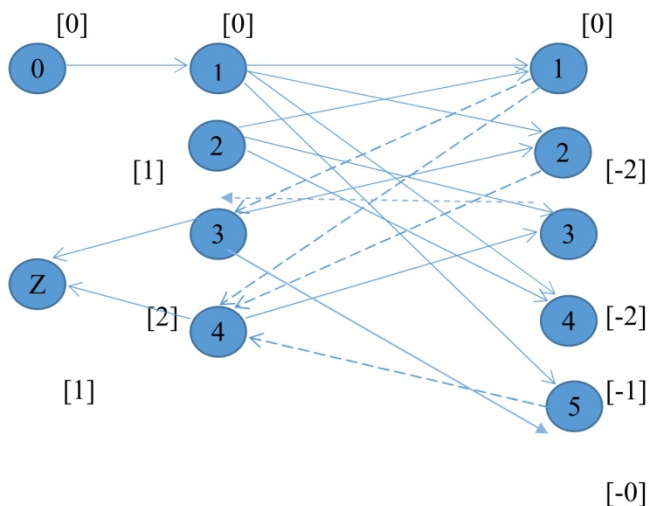
Рис. 3. Граф назначений
