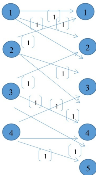
Рис. 1. Двудольный граф
