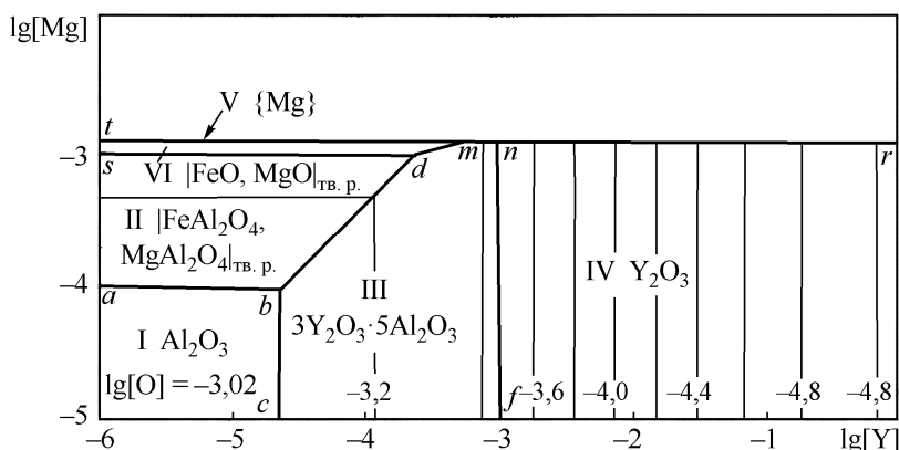
Рис. 2. ПРКМ системы \text{Fe}-\text{Y}-\text{Al}-\text{Mg}-\text{O} , T = 1600 °C, P_{\text{общ}} = 1 атм, [\text{Al}] = 0,005 мас. %
