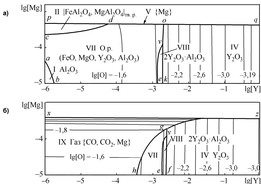
Рис. 3. ПРКМ системы \text{Fe}-\text{Y}-\text{Al}-\text{Mg}-\text{O} , T = 1890 °C, P_{\text{общ}} = 1 атм, [\text{Al}] = 0,005 мас. %:
