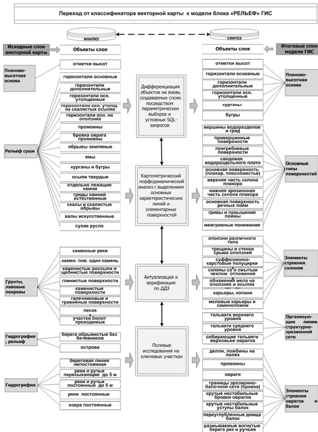
Рис. 1. Процедура построения модели рельефа в ГИС посредством осуществления семантических выборок, SQL-запросов, дешифровки ДДЗ, картометрии и полевых изысканий
