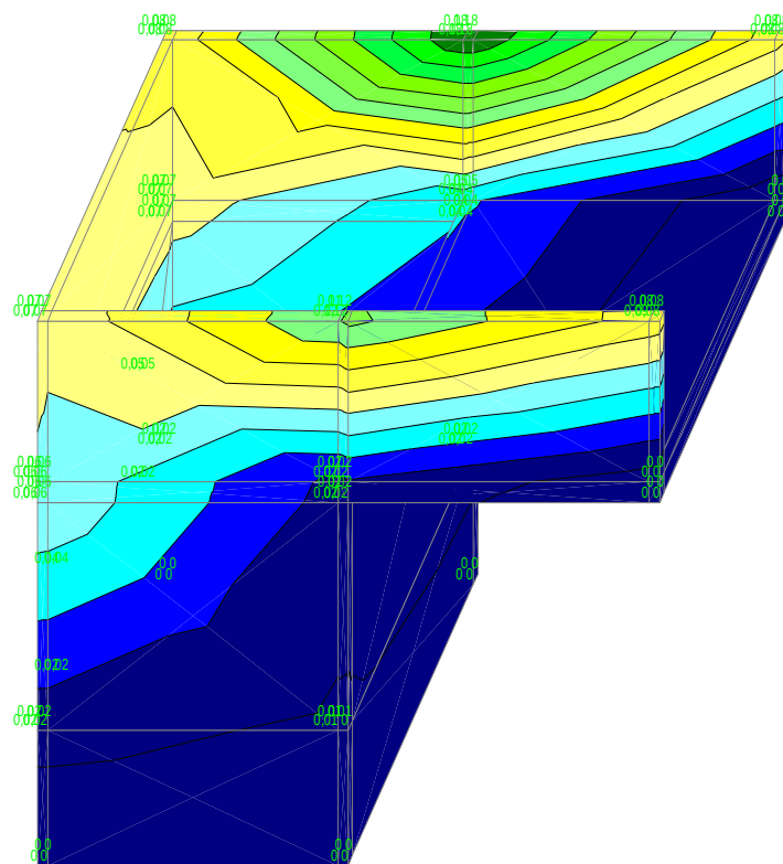
Рис. 2. Эпюра напряжений от динамических нагрузок
