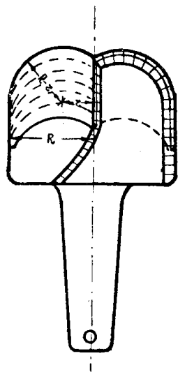
Рис. 3. Геометрия резца с равнопрочной режущей гранью
