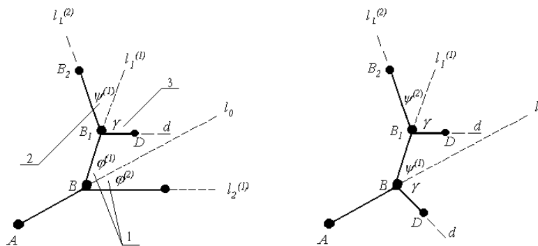
Рис. 6. До побудови моделі сегмента з піддеревами. Ліворуч: B – точка розгалуження; \phi^{(1)}, \phi^{(2)} – кути між материнським і дочірніми сегментами дендрита (маркер 1); \psi^{(1)} – проміжний кут (маркер 2); l_0, l_1^{(1)}, l_1^{(2)}, l_2^{(1)} – напрямки кроків; d – напрямок росту піддерева; \gamma – кут між кореневим і материнським сегментами (маркер 3). Праворуч: B – початок наступного кроку
