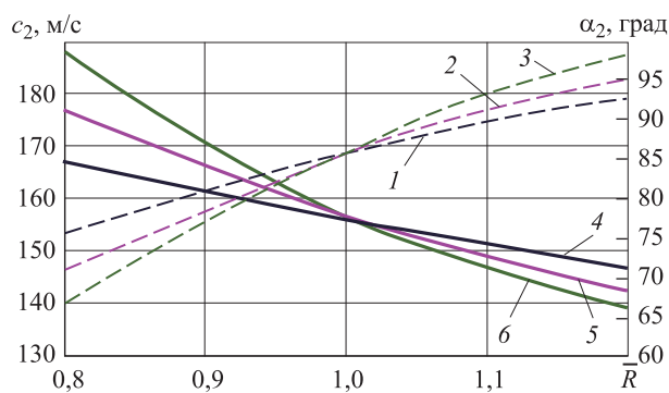
Рис. 7. Изменение углов \alpha_2 (1–3) и скорости c_2 (4–6) по радиусу R : 1, 4 — z = 0 ; 2, 5 — z = 0,5 ; 3, 6 — z = 1,0
