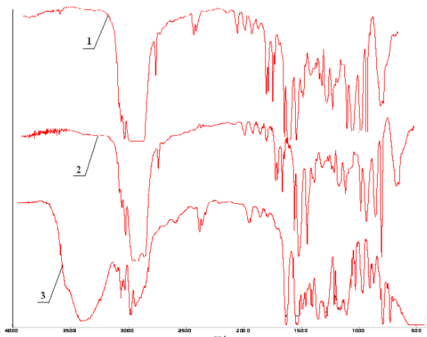
Рис. 1 – ИК-спектры пленок: 1 – ДСТ-30; 2 – ДСТ-30/МОПА; 3 – МОПА
